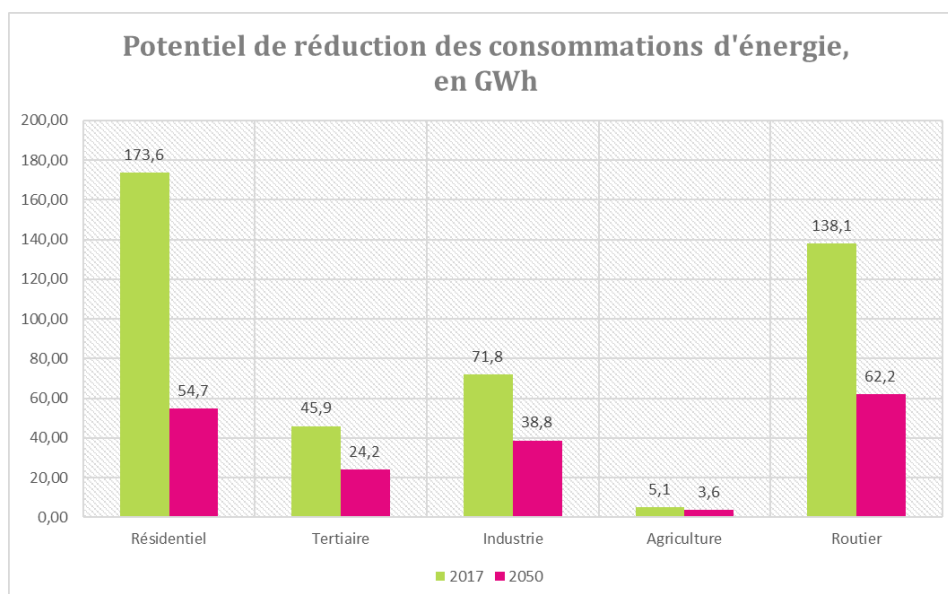
Figure 4 : évolution potentielle de la consommation d'énergie
